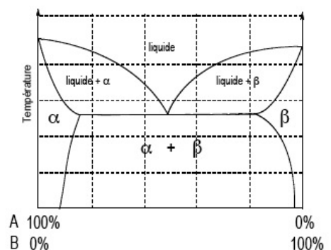
Diagramme des phases typique d'un eutectique
